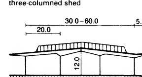
longitudinal section
